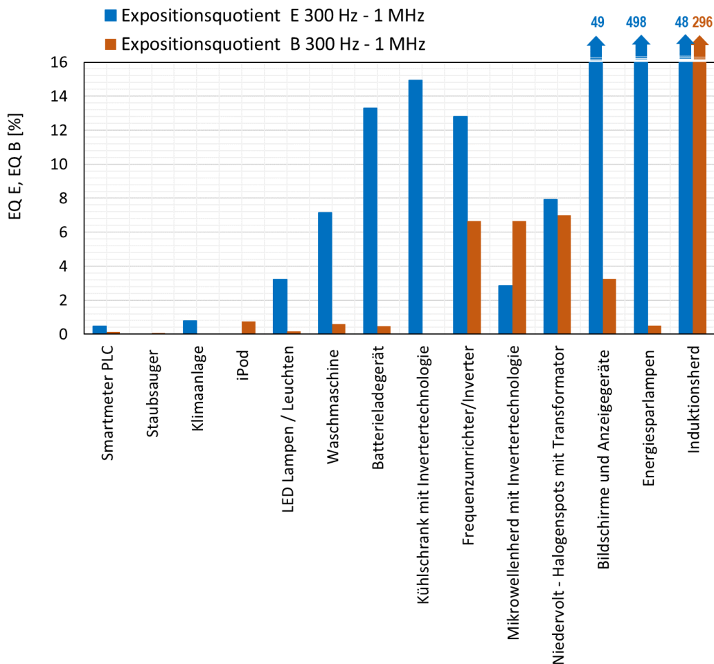
Abbildung 2 Durch Smart Meter Kommunikation verursachten Expositionsquotienten im Vergleich zu anderen Geräten im Haushalt (Viele Haushaltsgeräte verursachen zusätzlich wesentliche Anteile mit Frequenzen unterhalb von 300 Hz).
